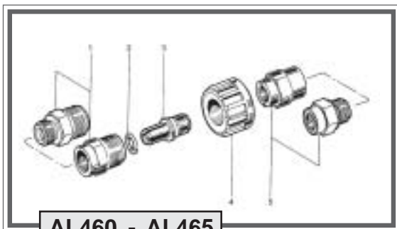
AL460 - AL465
