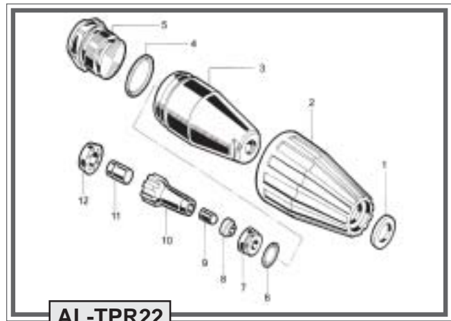
AL-TPR22
